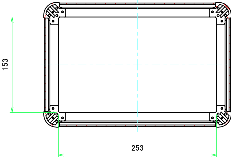
C-C ( 1 : 3.5 )
